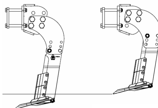
Głębokość MINIMALNA
